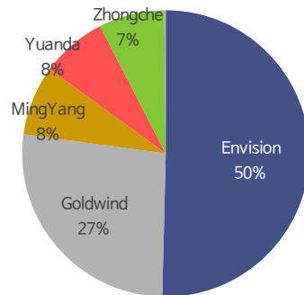
중국 풍력 터빈 수출 업체별 점유율 (2022)
