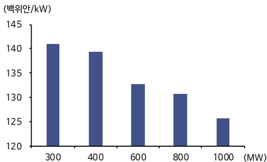
해상풍력 단지 설비 용량에 따른 투자 비용
