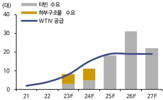
WTIV 수급 - 12MW 이상
