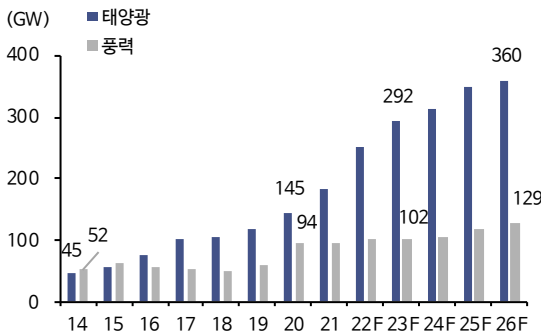
태양광, 풍력발전소 설치수요 추이
